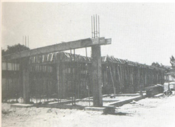
Construcción de la primera fase del Pabellón Polideportivo cubierto, en el recinto del Campo de Deportes «Ramón Díaz López».
