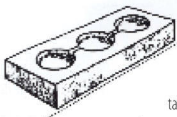
Molde abierto para fabricación de cospeles interconectados.
