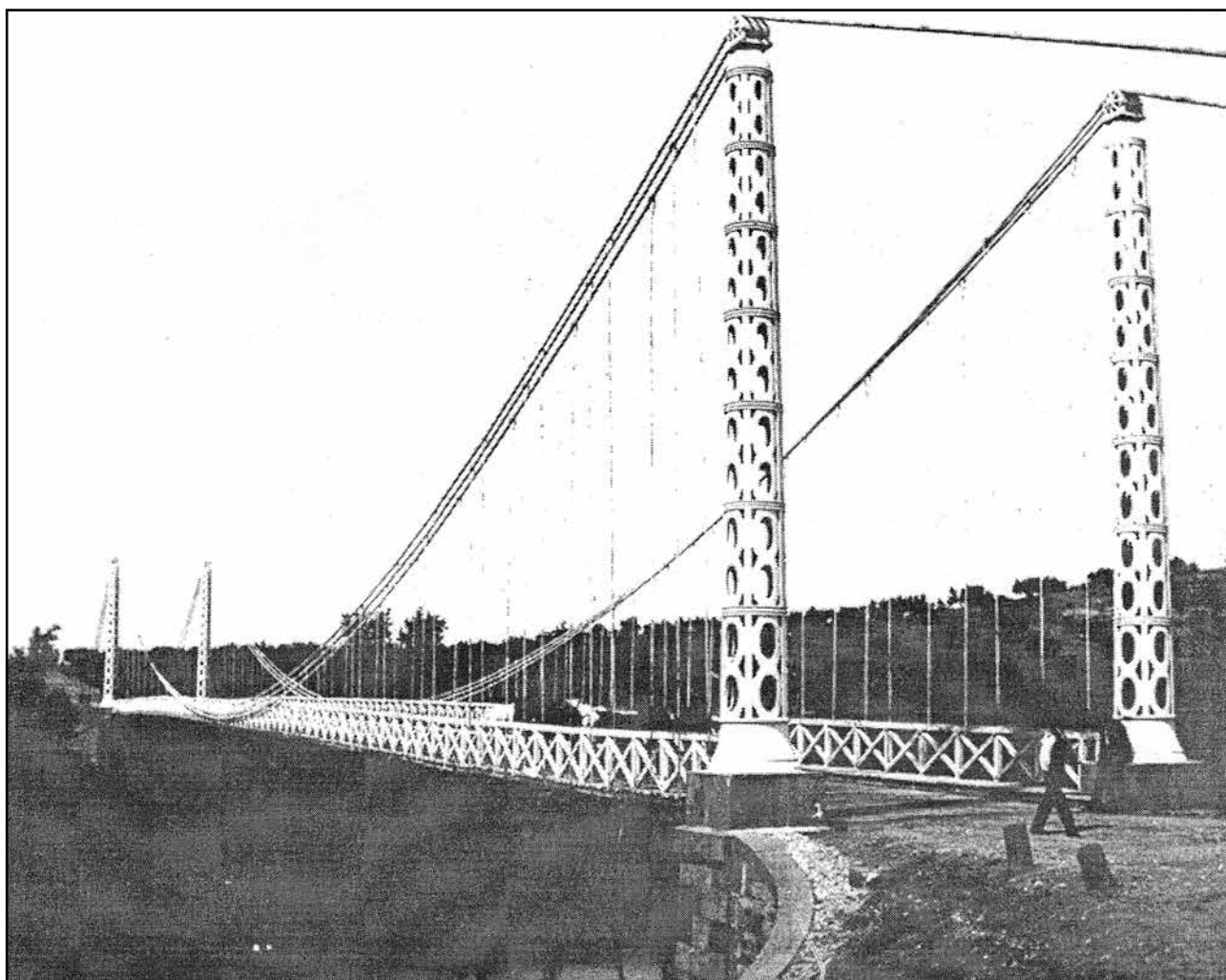
Puente colgante de Mengíbar. Libo de Feria año 1995. Artículo de Diego Galindo Ruiz
