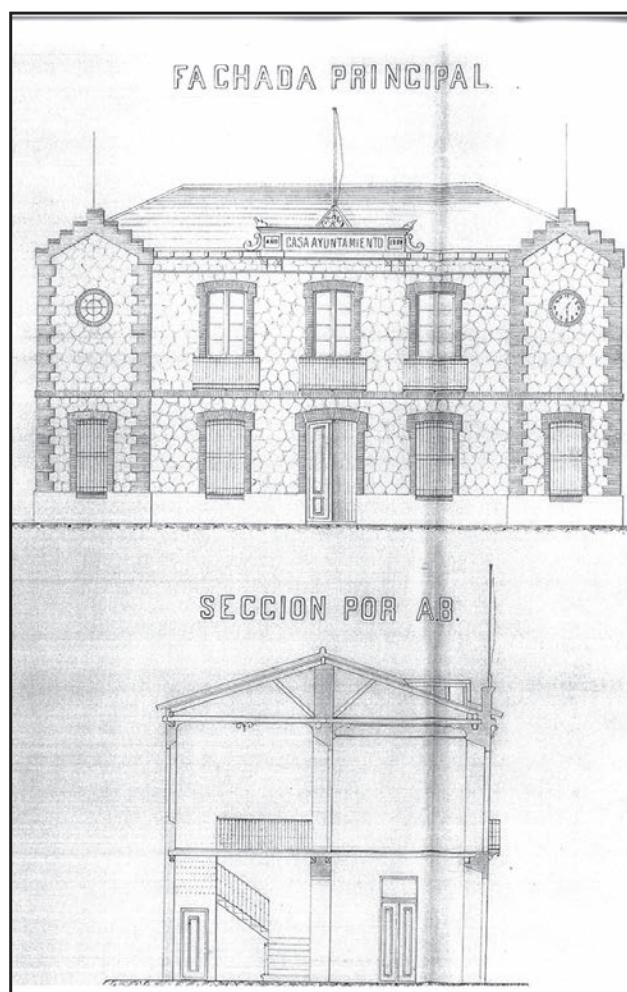
Fachada principal y sección del proyecto.
