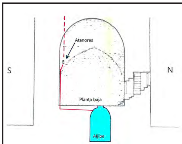
Recreación del sistema de almacenamiento de aguas pluviales procedentes de la terraza en el aljibe. Basado en un dibujo del proyecto de restauración de Ana Iglesias de 1982.
