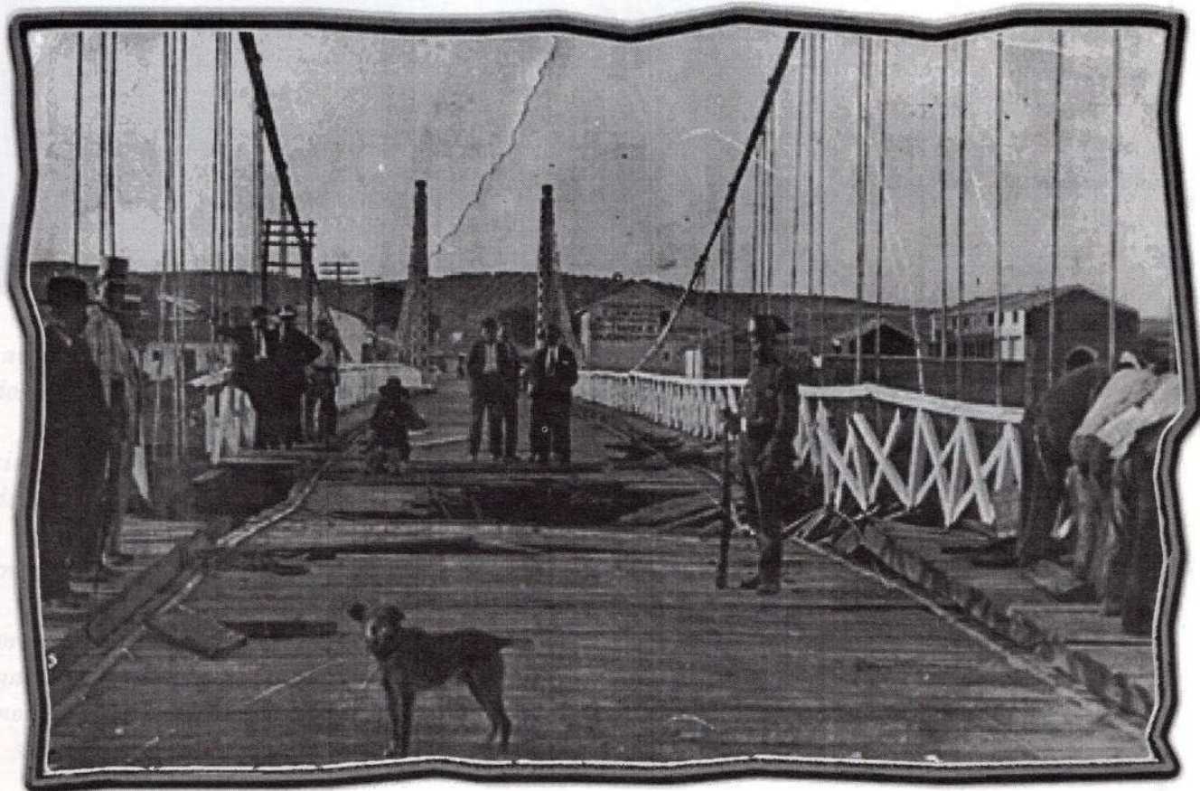
Estado del piso del Puente, después del accidente del 18 de agosto de 1930.
