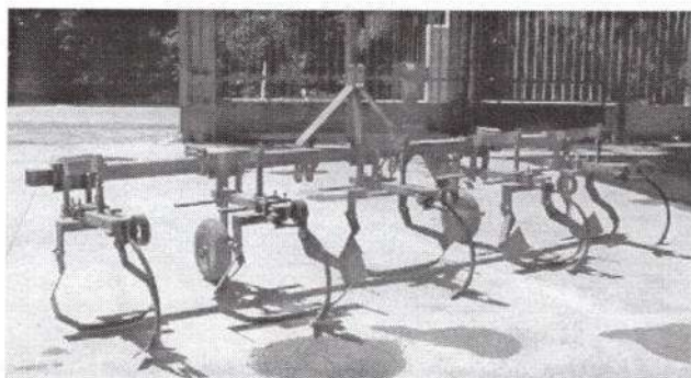
JUEGO DE CUCHILLAS ACOPLADAS A REGAVINA
