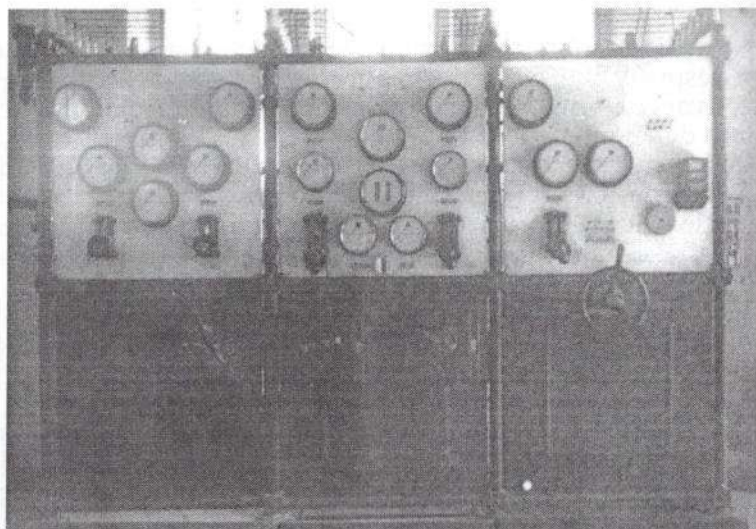
Cuadros de mandos de la Central Hidroeléctrica "La Purísima Concepción"
